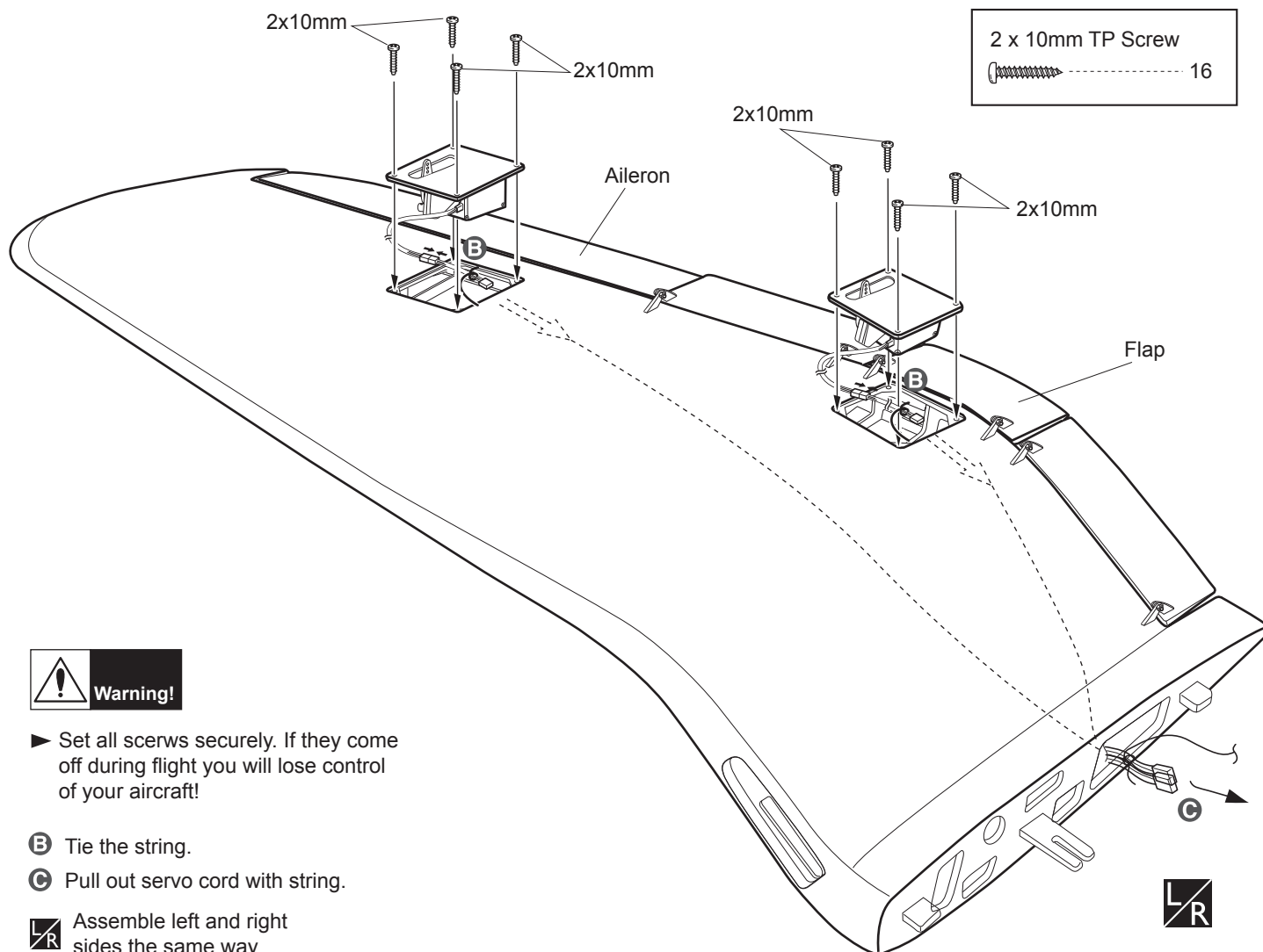
&lt; Right Wing &gt;
