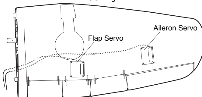
&lt; Left Wing &gt;
