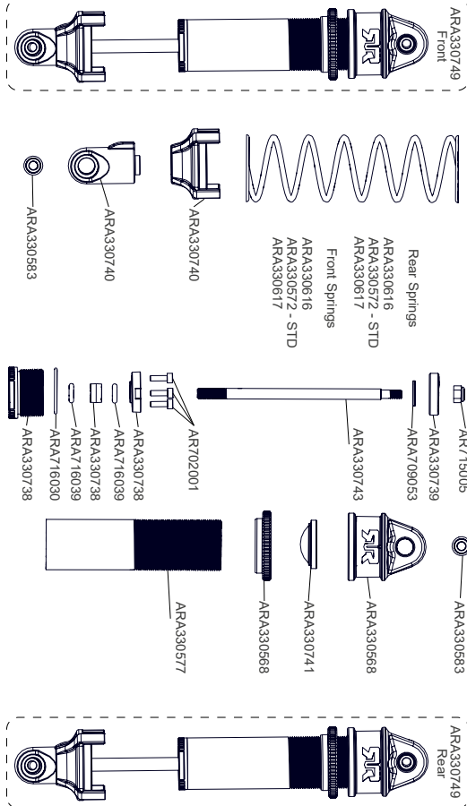
EXPLODED VIEW EXPLOSIONSANSICHT VUE ÉCLATÉE
